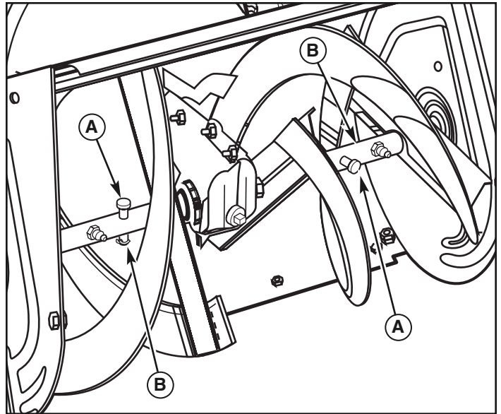
Remplacement des goupilles de cisaillement cassées Figure 22
