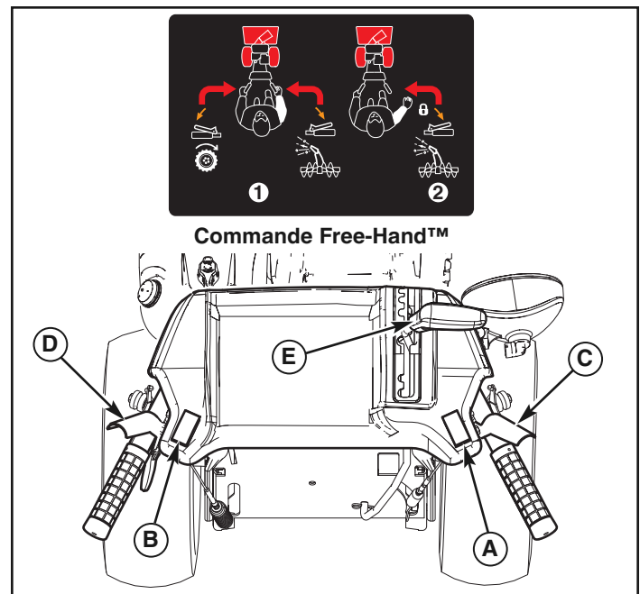
Leviers de commande
