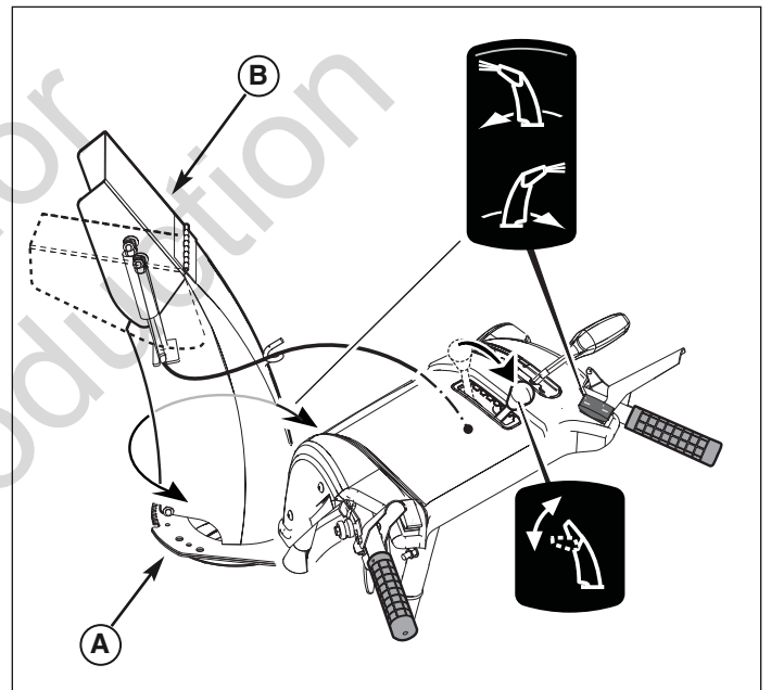
Goulotte et déflecteur d'éjection
