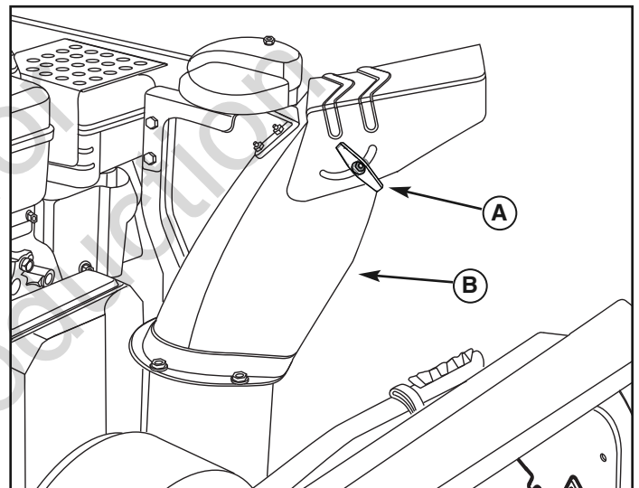
Réglage de l'angle du déflecteur d'éjection
