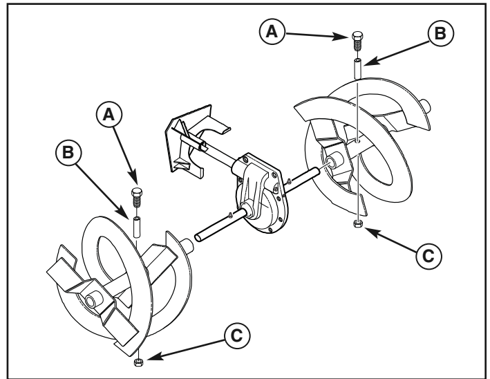
Remplacement de la goupille de cisaillement cassée Figure 20
