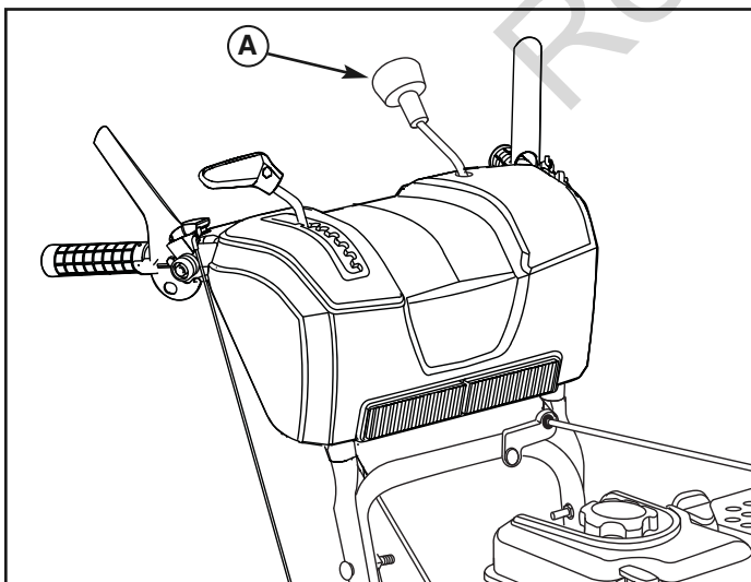
Réglage de la rotation du conduit d'éjection
